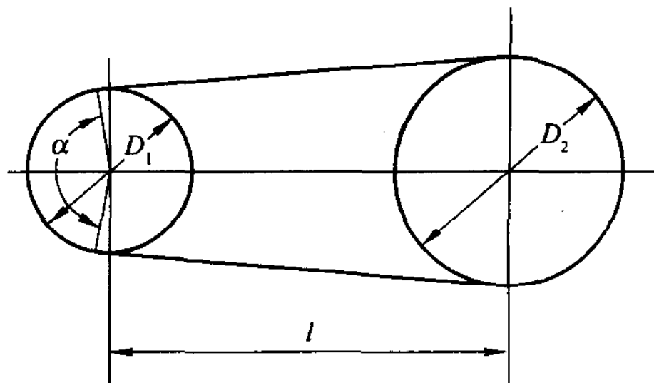
图 1-1 带传动
