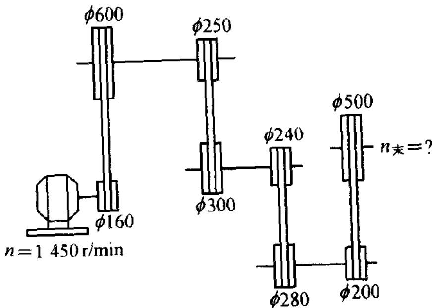
图 1-2 由几对带轮组成的带传动
