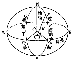
图 1-5 大地坐标系
