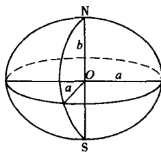
图 1-3 旋转椭球体
