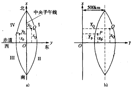
图 1-10 高斯平面直角坐标系
