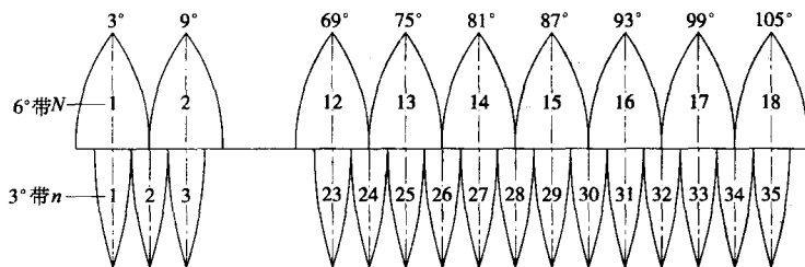
图 1-9 6°带投影与 3°带投影的关系
