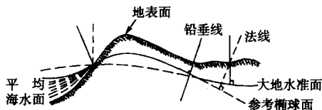
图 1-2 大地水准面
