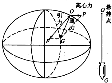
图 1-1 铅垂线方向
