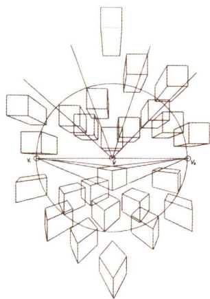
图 1-10 透视规律图
