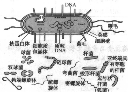
图 2-1 细菌结构示意图
