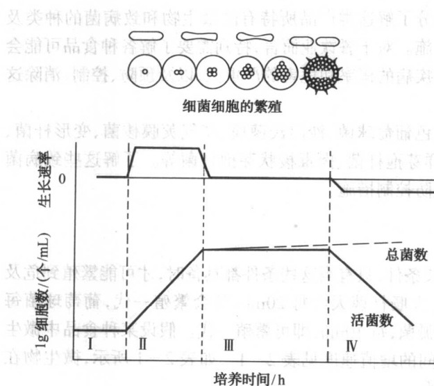
图 2-2 微生物的典型生长曲线
