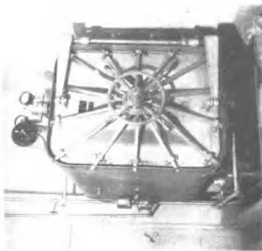
单扉式高压消毒柜
