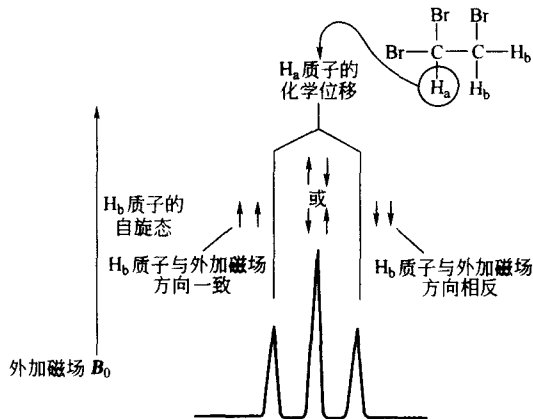
图 1.12 ^1\text{H} NMR 中质子的耦合示例
