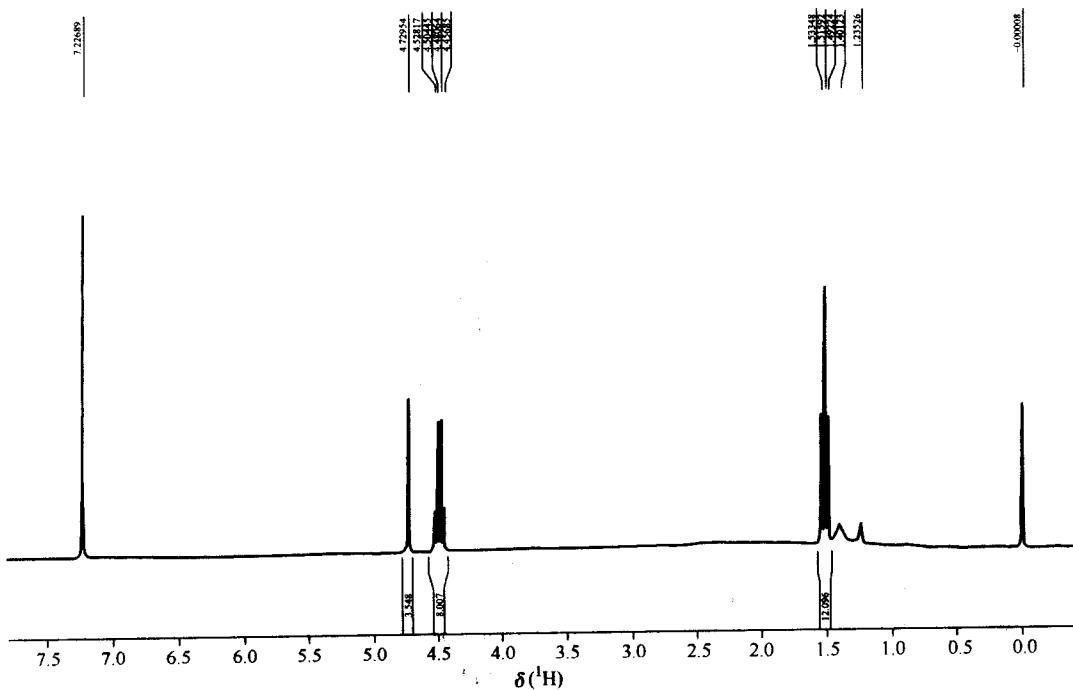
图 1.10 分离后纯品的 ^1\text{H} NMR 谱 ( \text{CDCl}_3\text{-CS}_2 , 300 MHz)
