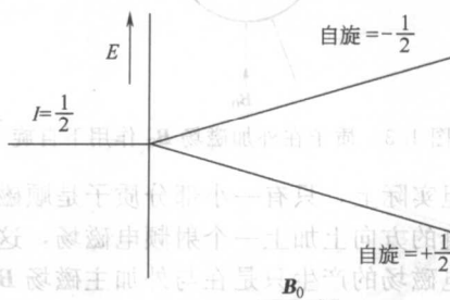
图 1.2 质子在磁场 B_0 下的两个能级
