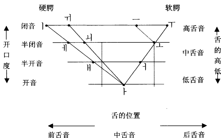
元音三角图
