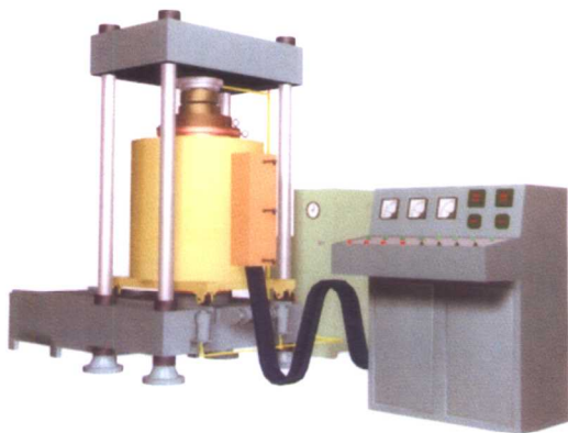
RYL80-36 井式可控气氛烧结压机
