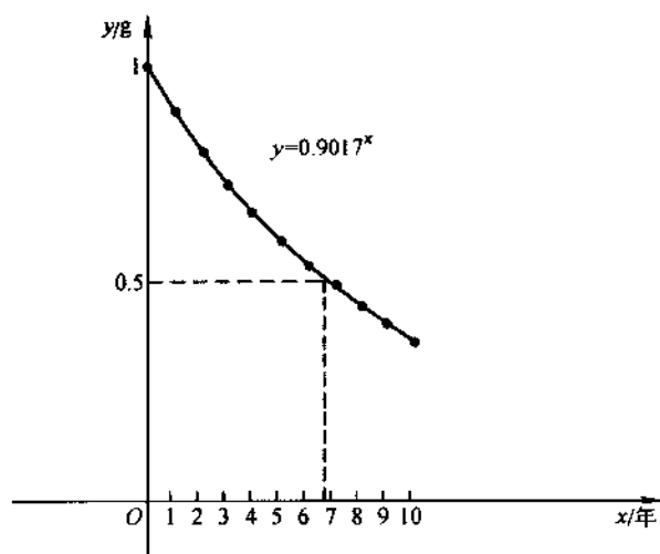
放射性物质镭 - 228 的半衰期约为 6.7 年
