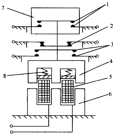
图 1-1 接触器结构简图
