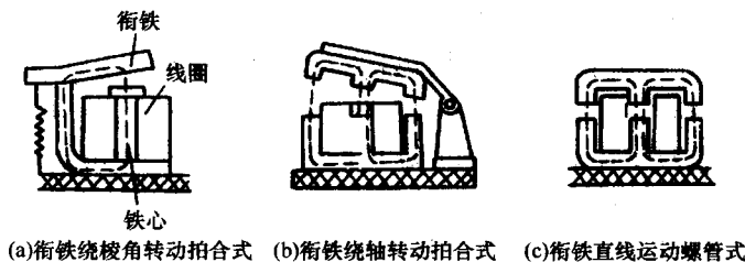
图 1-2 接触器电磁系统的结构图
