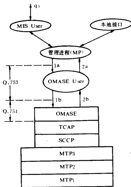
图 1.5 No. 7 信令点内部结构模式
