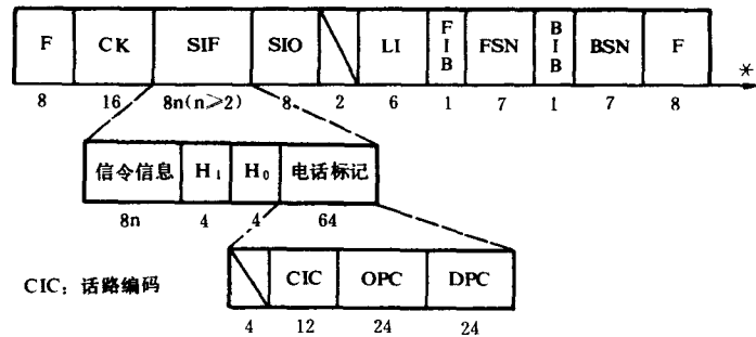
图 2.6 电话消息信号单元格式
