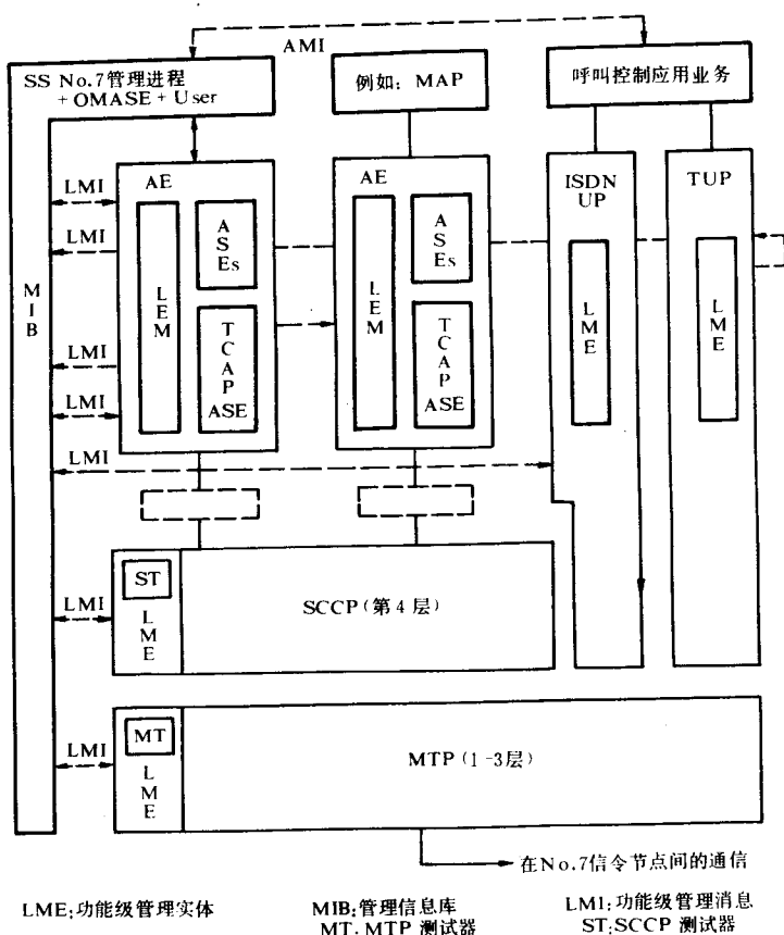
图 1.4 No. 7 信令的 OMAP 模式
