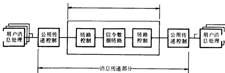
图 1.1 No. 7 信令系统的基本功能结构
