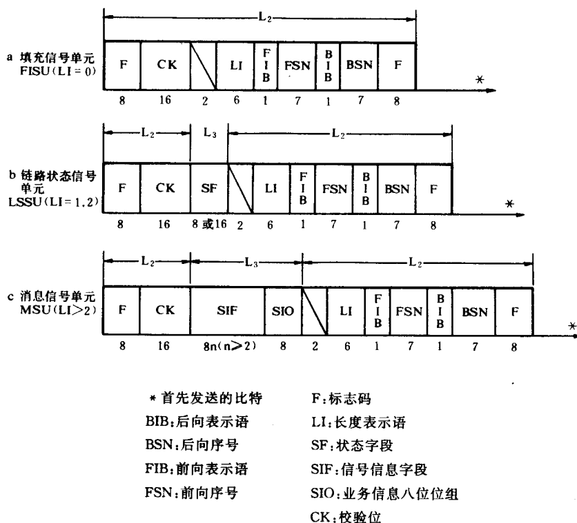
图 2.1 信号单元格式
