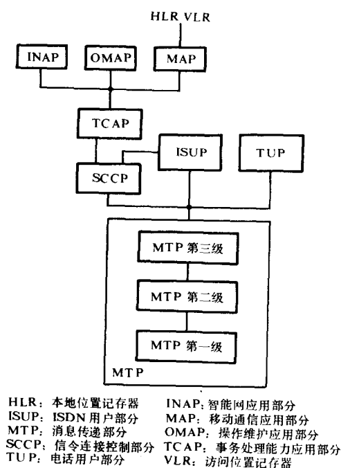
图 1.3 No. 7 信令系统的规程结构图
