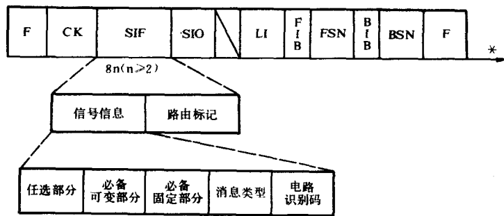
图 2.7 ISUP 信号单元格式
