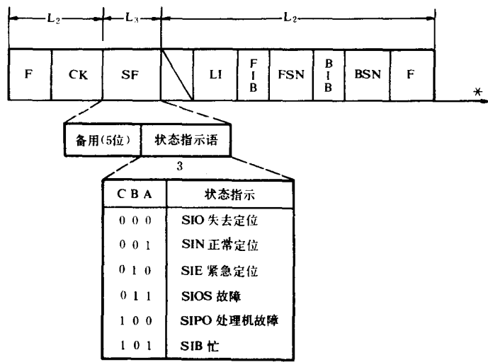
图 2.2 链路状态信号单元
