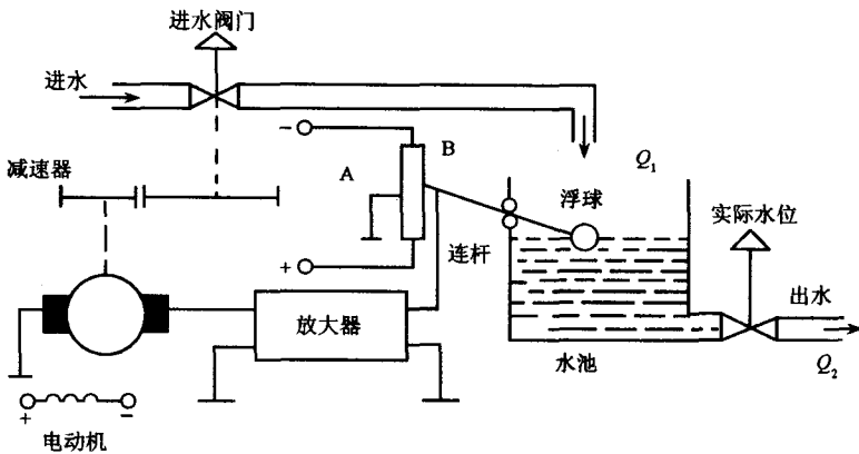
图 1-5 水池水位控制系统原理示意图
