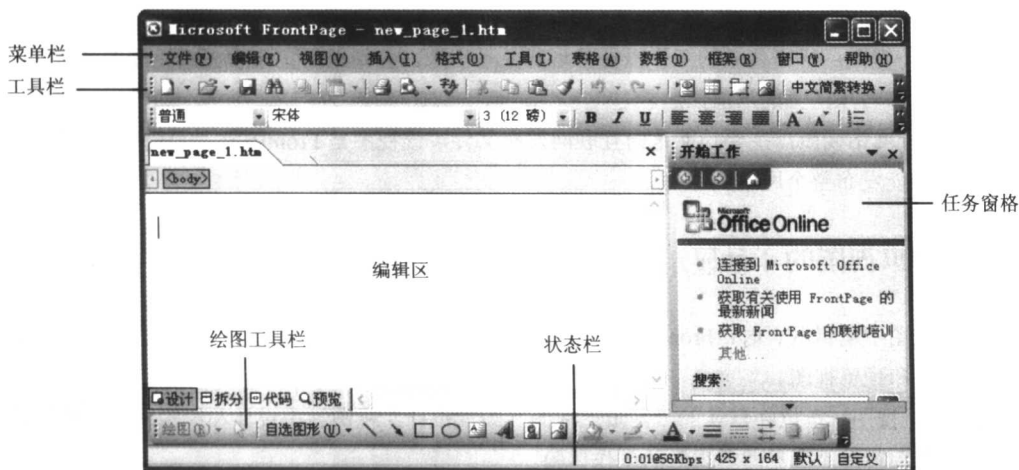
图 1.3.1 FrontPage 2003 窗口
