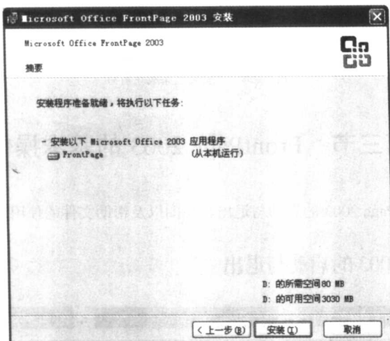
图 1.2.6 “摘要”窗口
