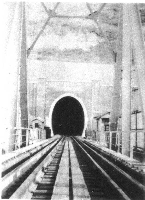
▲ 焦枝铁路邙山隧道
