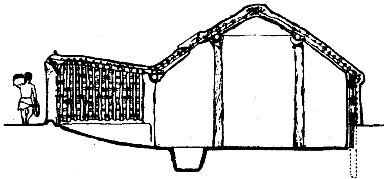
图三 庙底沟遗址第 302 号房址复原图
