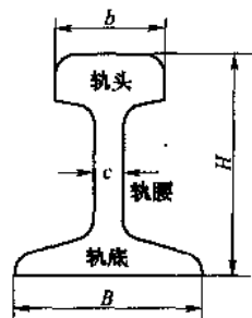
图 1-1 钢轨断面
