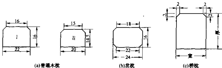
图 1-5 木枕尺寸 (单位: cm)
