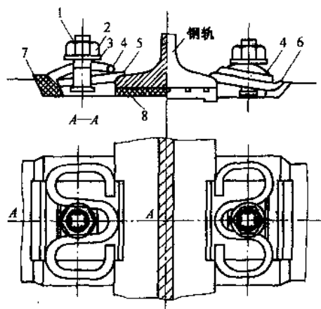
图 1-7 \omega 形弹条扣件
