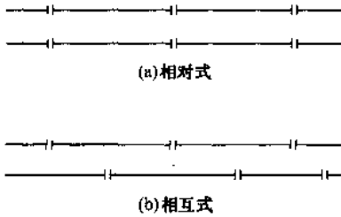
图 1-3 钢轨接头相互位置
