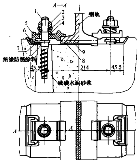
图 1-6 70 型扣板式扣件 (单位: mm)
