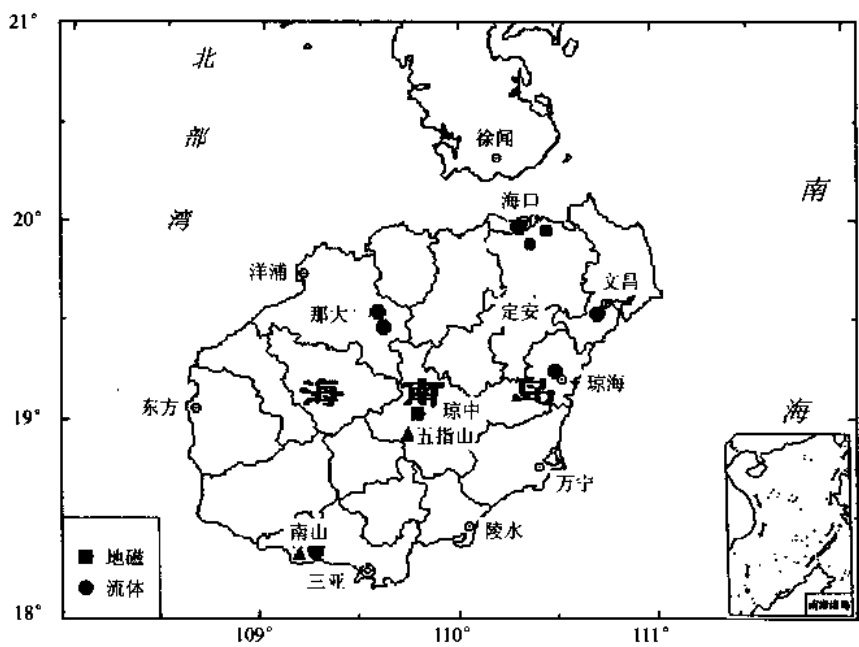
图 1-3-2 海南省地震前兆台站分布图
