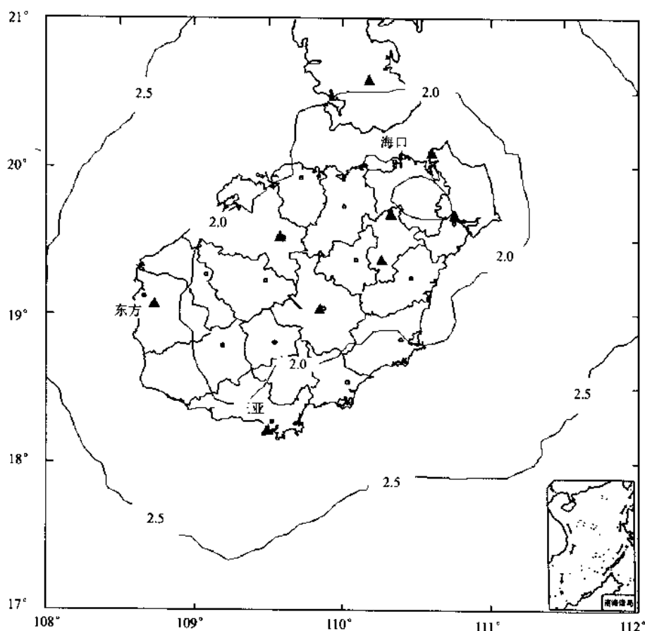
图 1-3-3 海南省地震监控能力图
