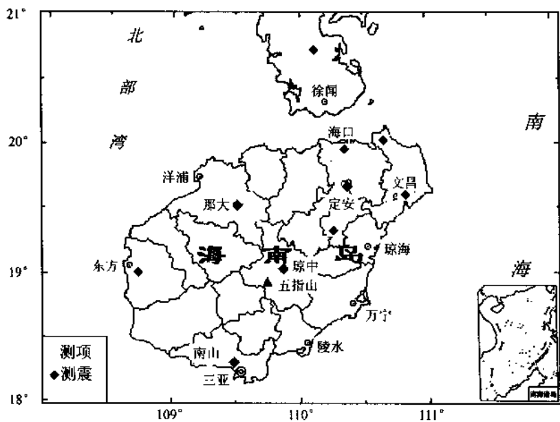
图 1-3-1 海南省测震台网分布图
