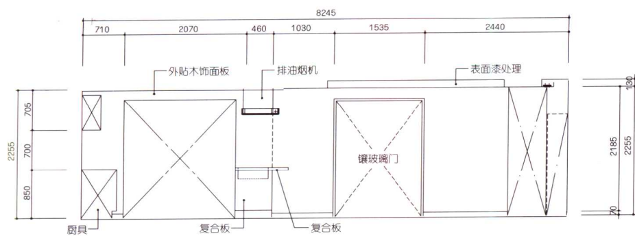
立面图
