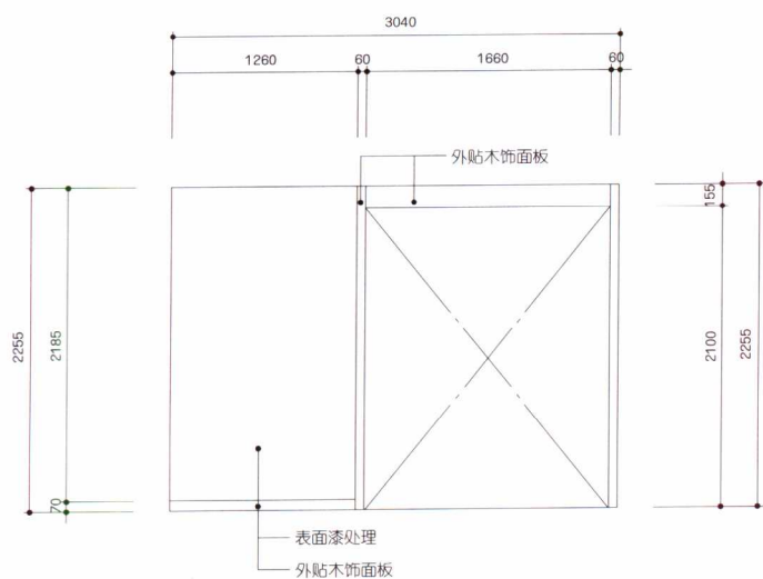
立面图
