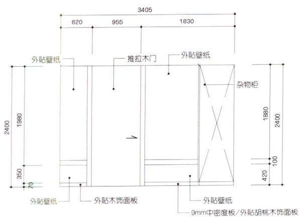
立面图
