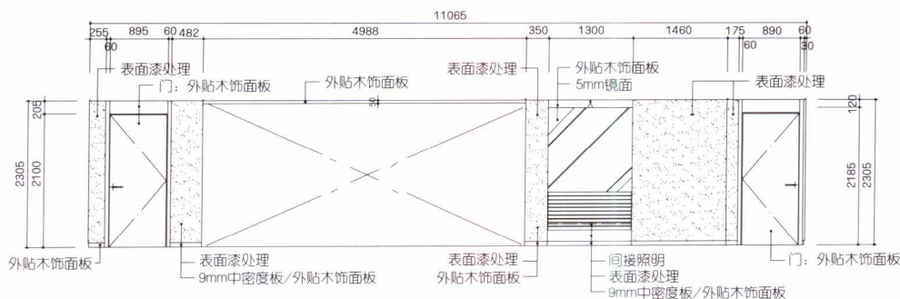
立面图
