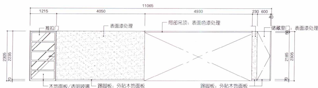
立面图
