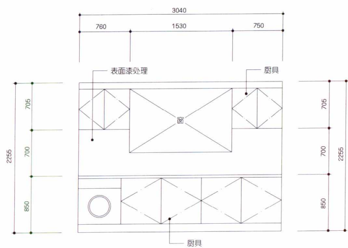
立面图
