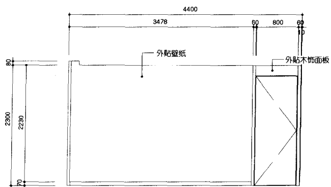
立面图
