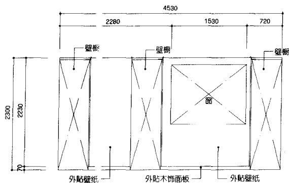
立面图
