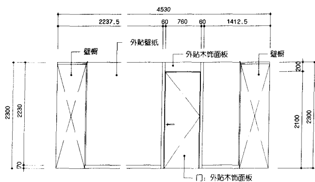
立面图
