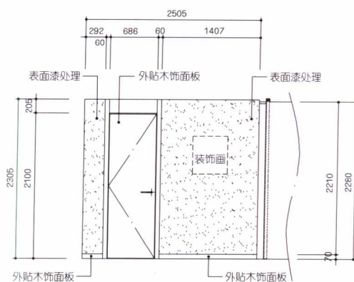
立面图
