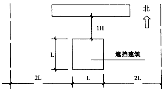
图 2.2.3-3 塔式建筑遮挡建筑
