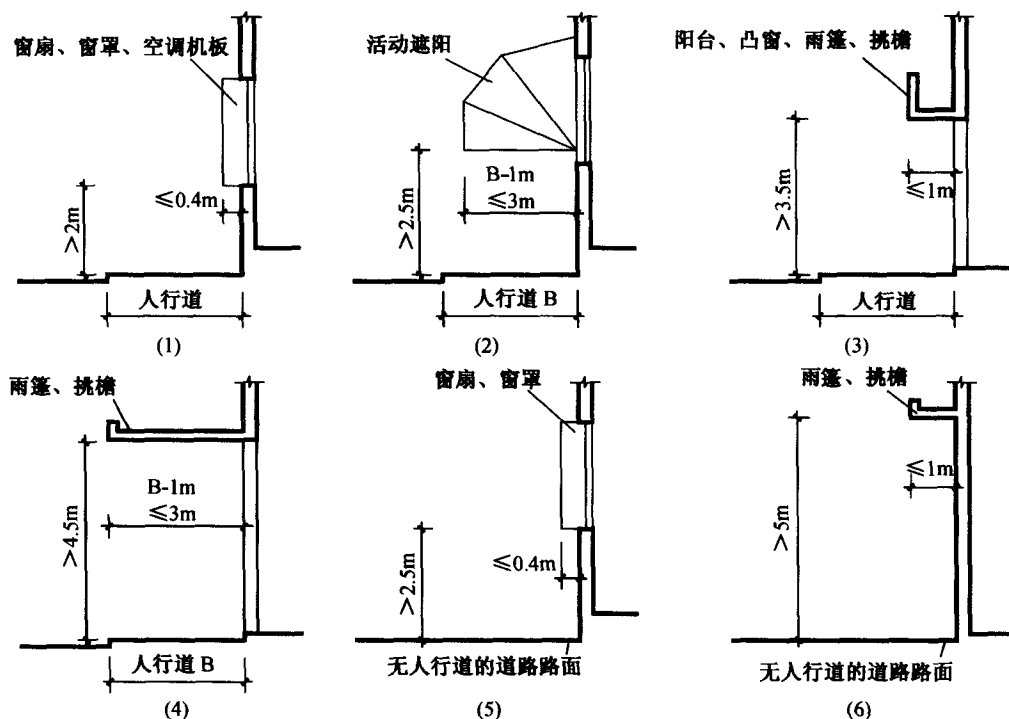
图 2.1.2-1 允许突出道路红线上空的建筑突出物
