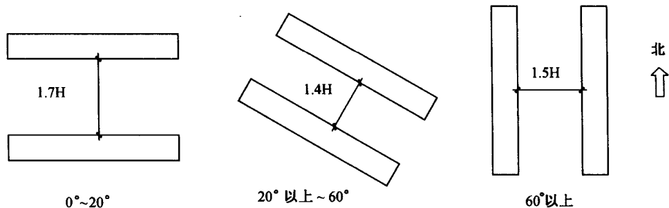
图 2.2.3-2 板式建筑遮挡建筑
