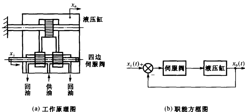
图 1-8 液压伺服系统
