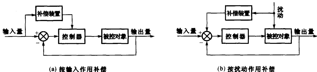
图 1-9 复合控制系统
