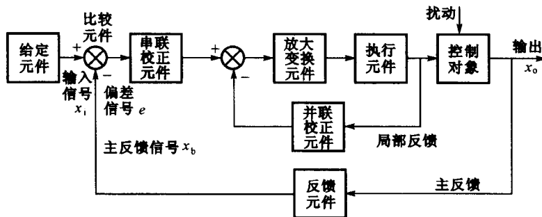
图 1-10 典型闭环控制系统的职能方框图
