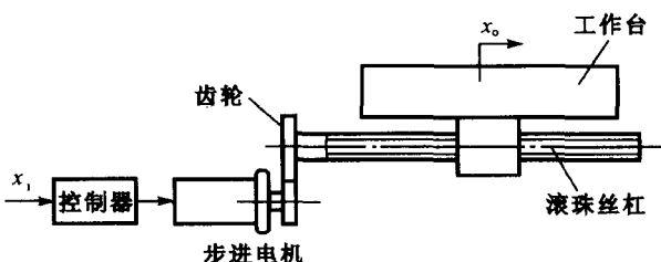
图 1-5 数控线切割机的进给系统
