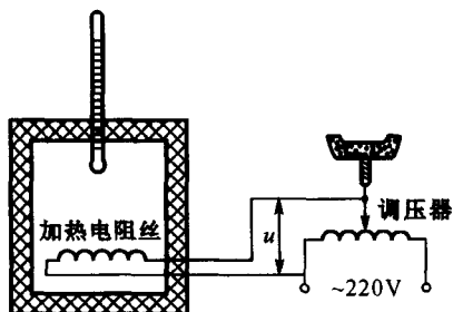
图 1-2 人工控制恒温箱
