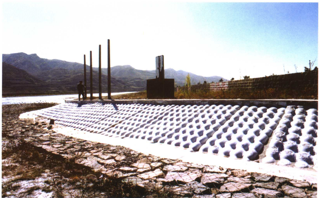
正在施工中的汾河上游滚水坝
