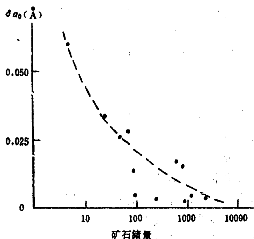
图1-2 矽卡岩型铁矿规模(储量以百万吨计)与磁铁矿的 \delta\alpha_0 的相关性 (M.З. Кантор)
