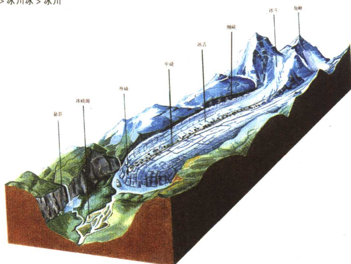
大型冰川 - 山谷冰川模式图
