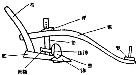
曲辕犁详图
