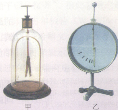
图 1.1-2 验电器和静电计
