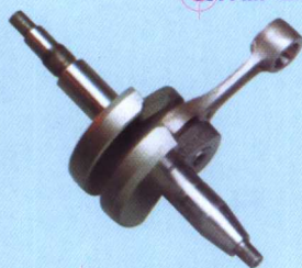
小型汽油机曲轴连杆组合
