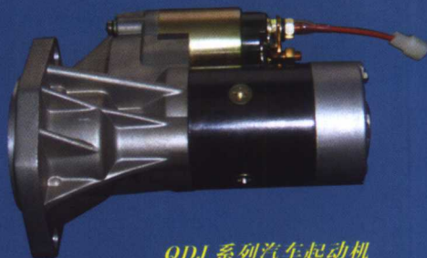
QDJ 系列汽车起动机
