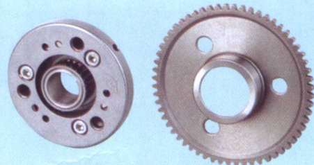
152QMI 适用于豪迈GY6125型发动机
