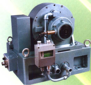
GW型电涡流测功机
