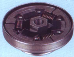
离心离合器
