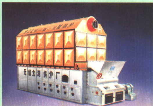
SZL 系列 6-15 t/h 锅炉
