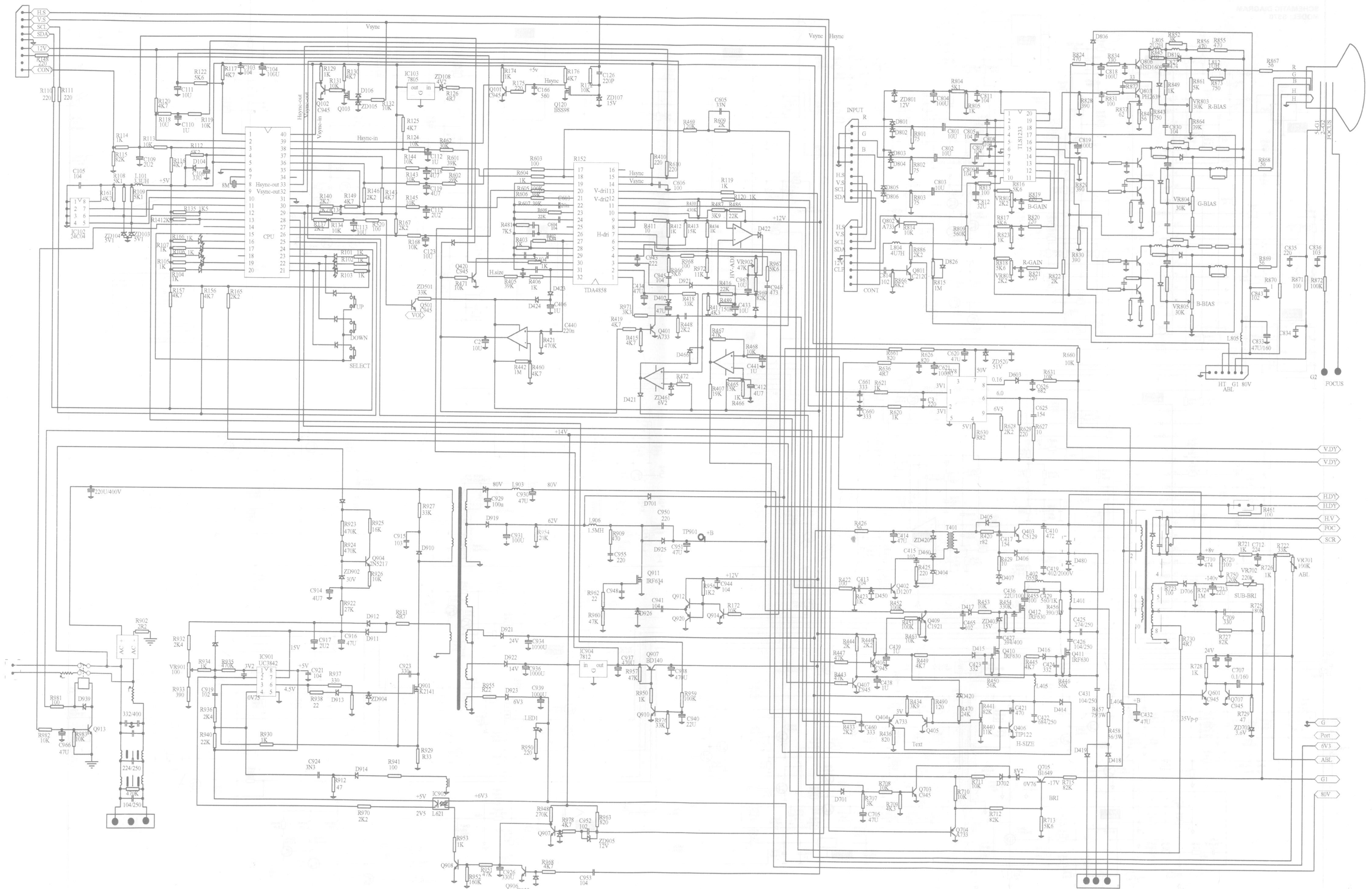
长城 CH-1527 彩色显示器整机电路
