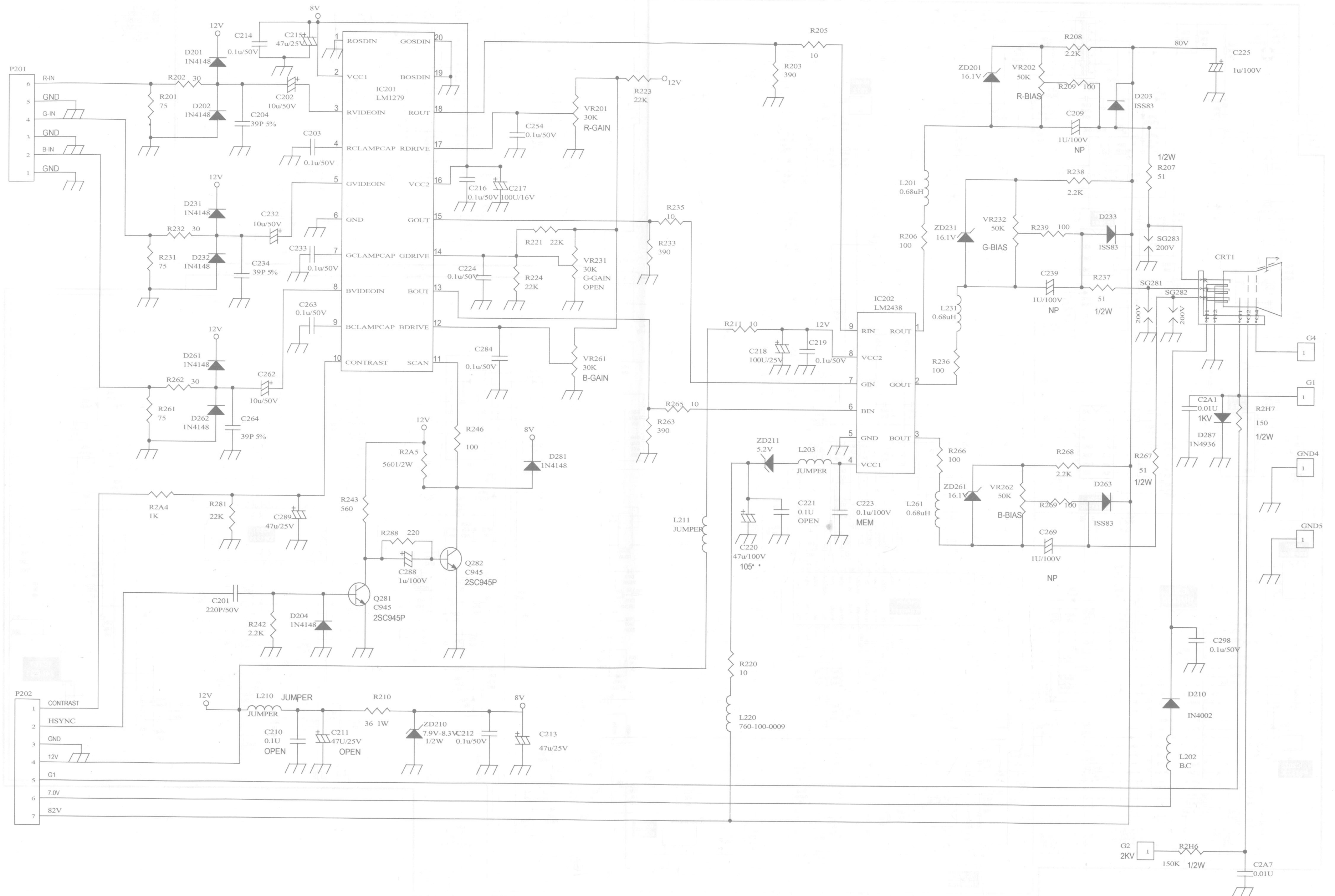
华冠 ( EMC ) X558 彩色显示器视频放大电路
