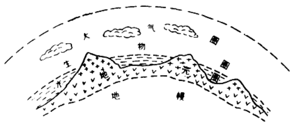
图 1-1-1 地球表面圈层结构示意
