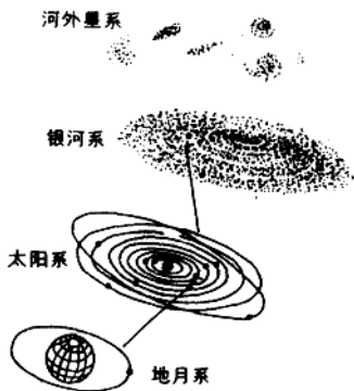
图 1-1-4 宇宙中不同级别的天体系统
