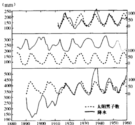
图 1-1-5 太阳黑子与年降水量的相关性
