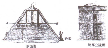
剖面图
