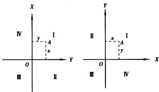
(a) 测量坐标系
