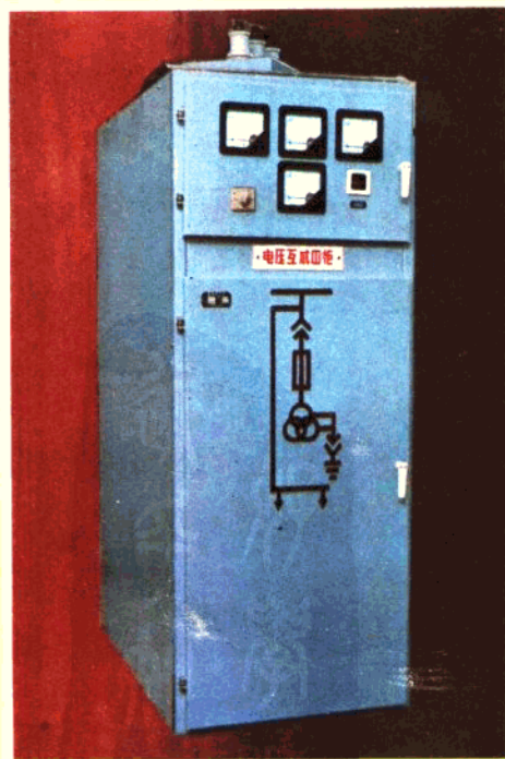
GC—1 手车式高压开关柜
