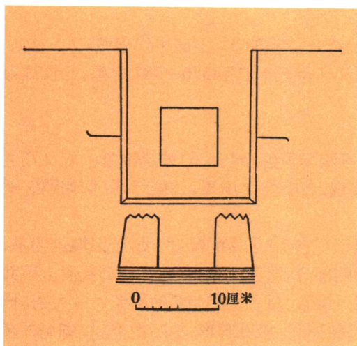
图 4-1-2 统万城一号马面竖坑平、剖面图(考古.1981.3:228)
