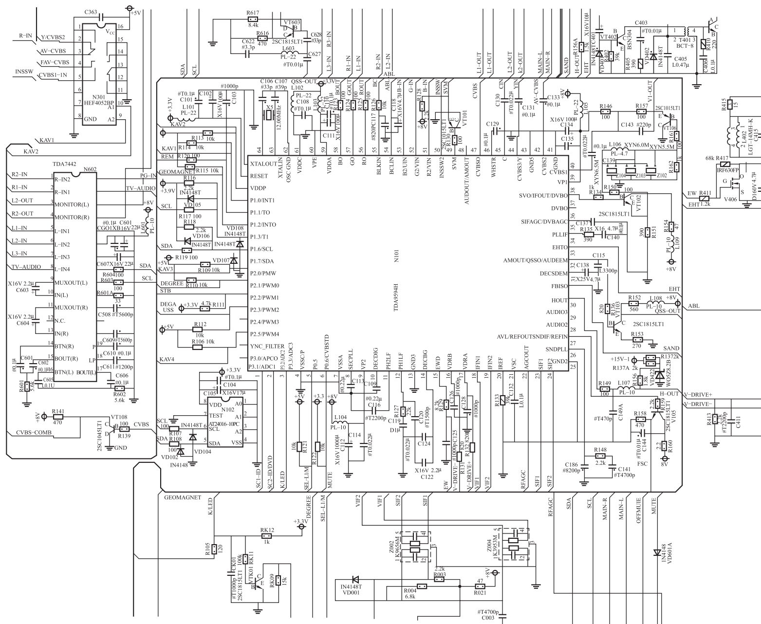
图 1-5 长虹 CH-20 机芯电视机超级芯片电路
