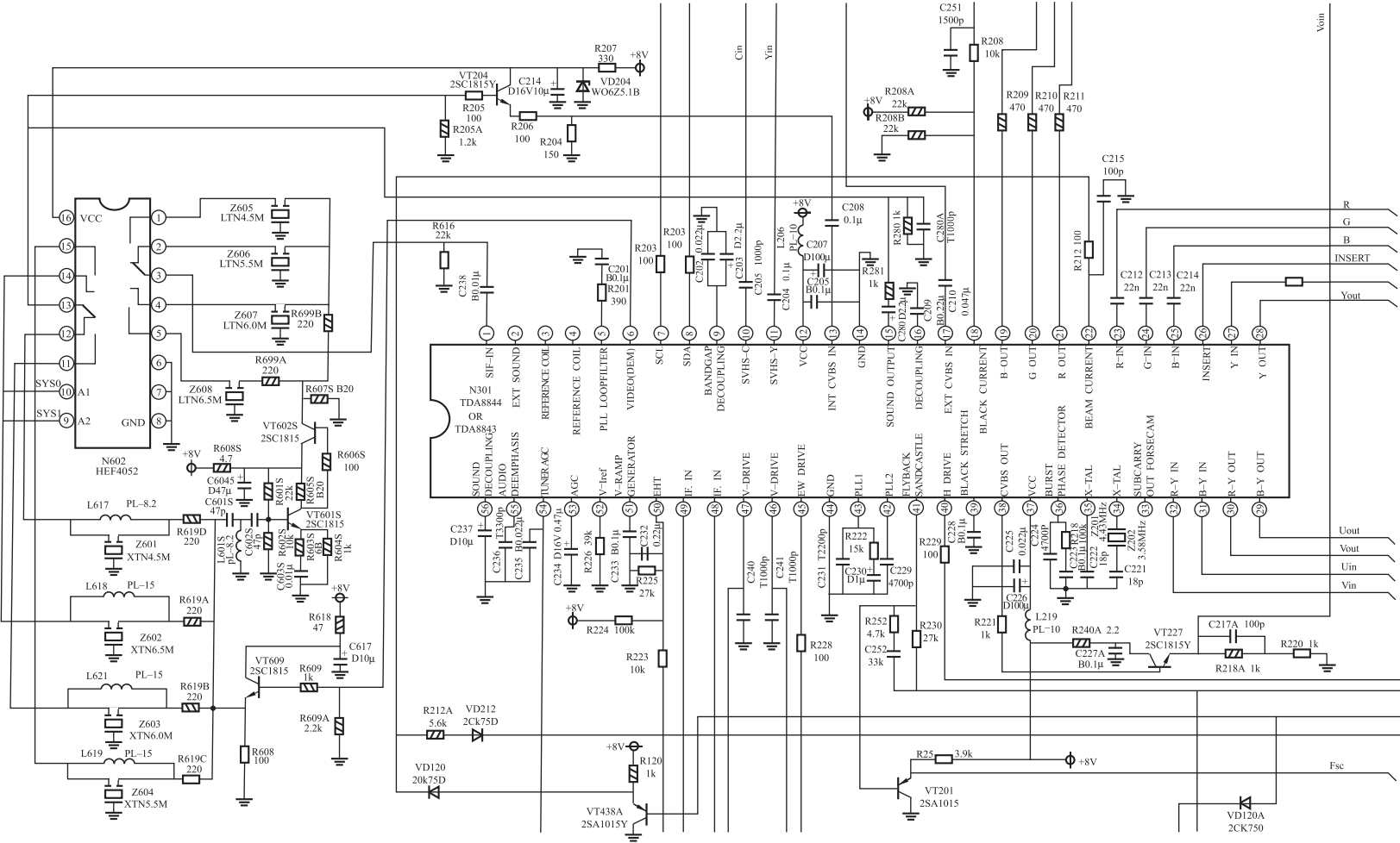
图 1-1 长虹 CH-10DR 机芯 (H29D80) 电视机单片小信号处理电路
