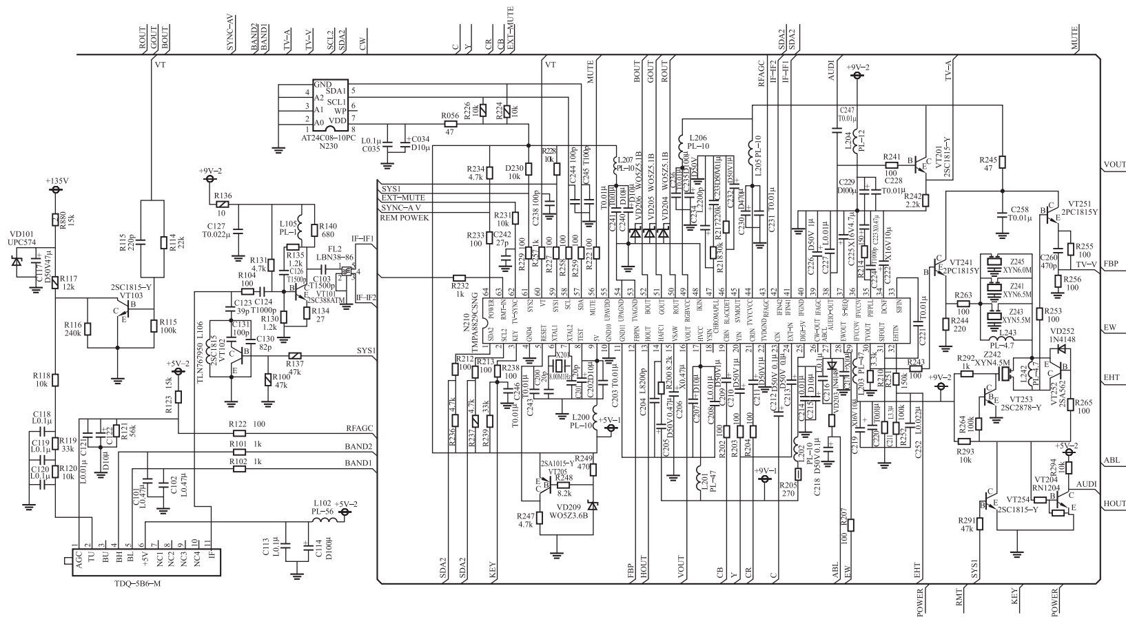
图 1-8 长虹 PF2991E 电视机超级芯片电路
