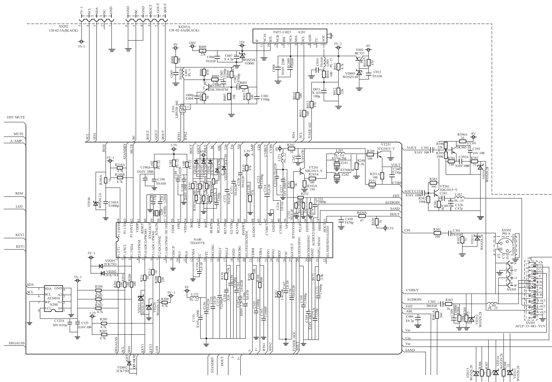
图 1-3 长虹 CH-16 机芯 (PF21156) 电视机超级芯片电路
