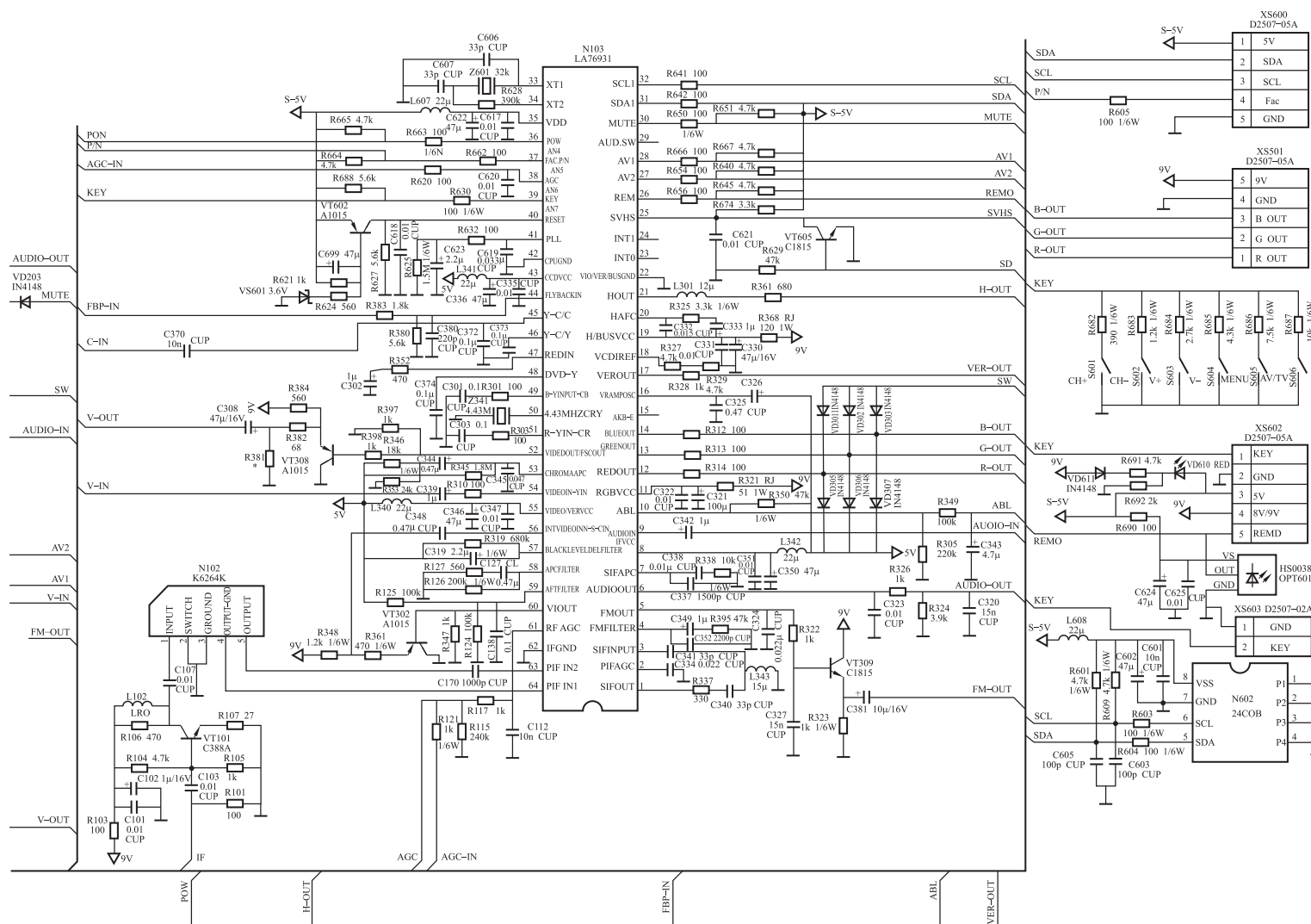
图 2-1 康佳 LA76931 超级芯片电路
