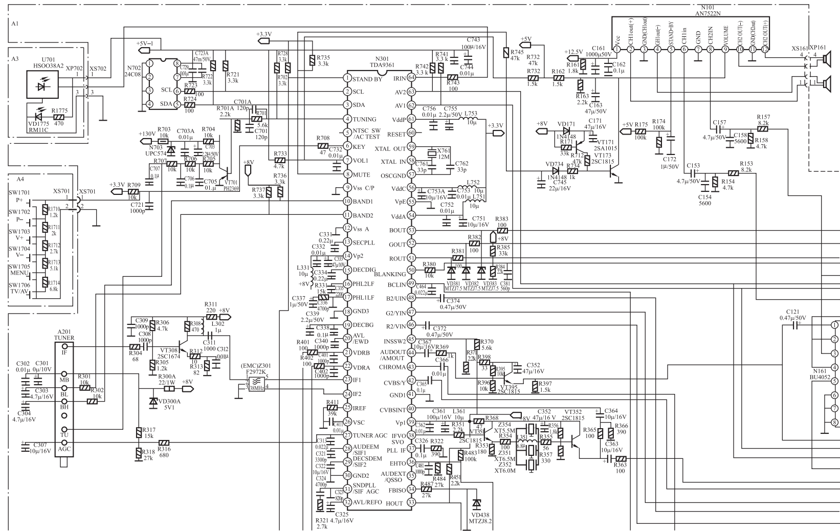
图 1-6 长虹 PE3495AST 电视机超级芯片电路
