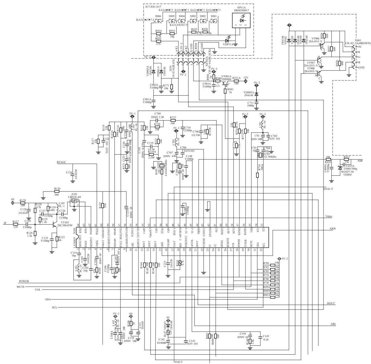
图 1-4 长虹 CH-18B 机芯 (PF21300) 电视机超级芯片电路
