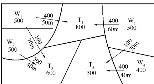
图 1-8 土方调配图
