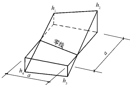
图 1-6 两挖和两填的方格
