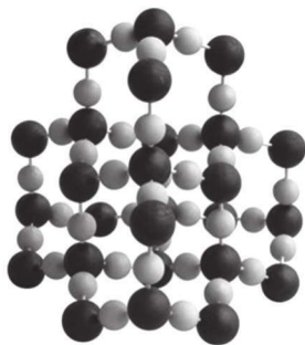
图解分子结构模型
