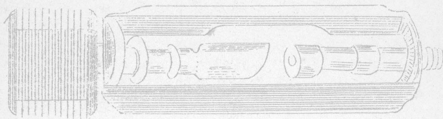
图7 空气自冷式X线管
