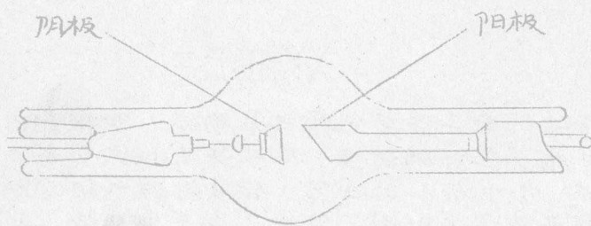
图2 热阴极X射线管
