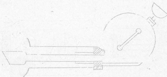
图8 水冷式X射线管
