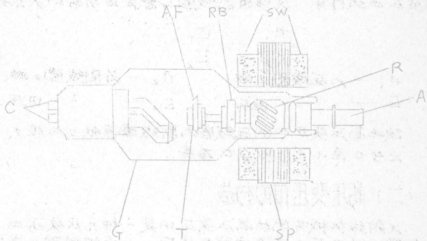
图9 旋转阳极式X射线管
