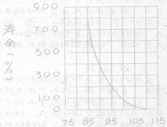
图3 灯丝加热与其寿命关系曲线
