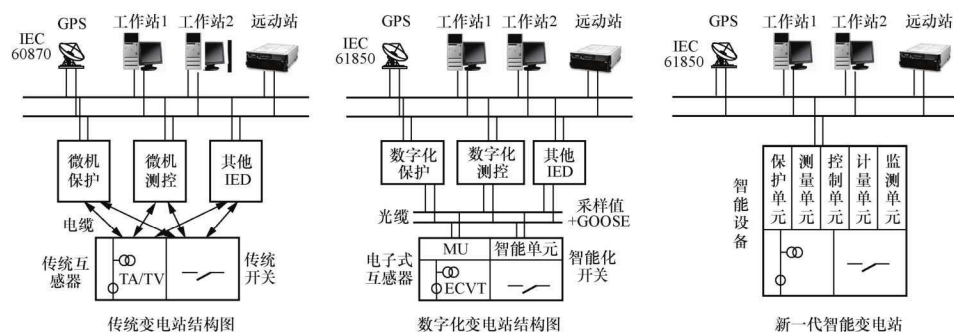
图 1-2 各阶段变电站网络结构对比图
