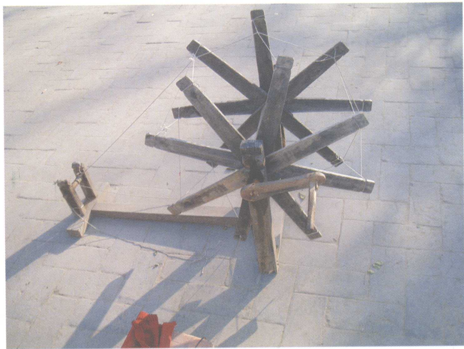
图11 纺花车
