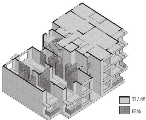
图0-5 剪力墙结构建筑示意图
