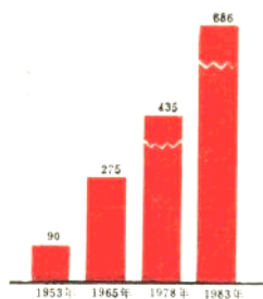
通车里程 公里
