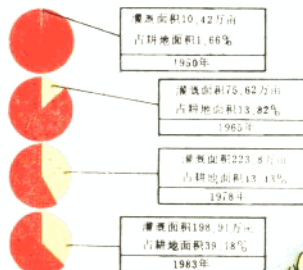
灌溉面积 (万亩)
