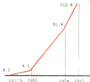
农业机械总动力 (万马力)
