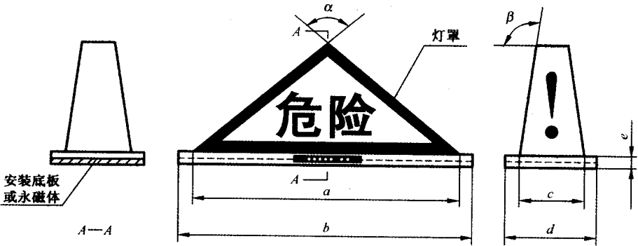
图 1 A 型标志灯
