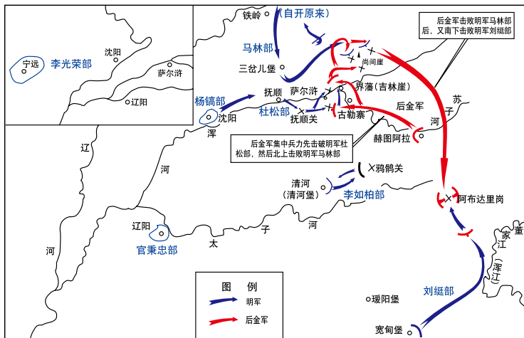
● 萨尔浒之战作战经过示意图
