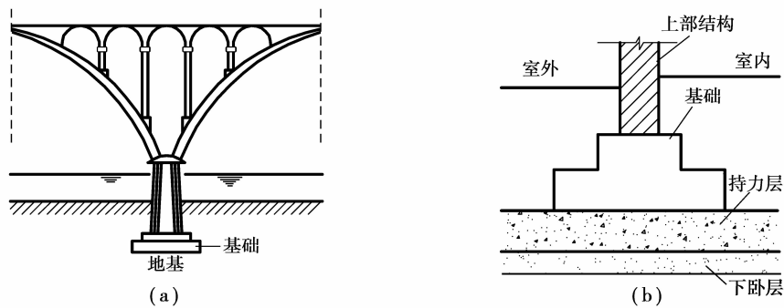
图 0.1 地基与基础
