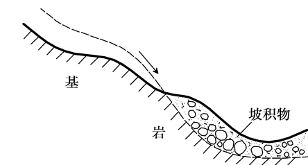
图 1.2 坡积土
