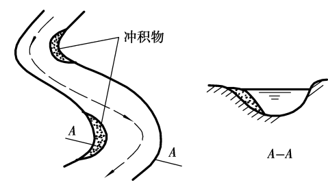
图 1.4 冲积土
