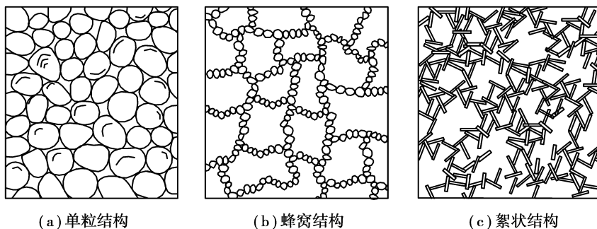
图 1.5 土的结构
