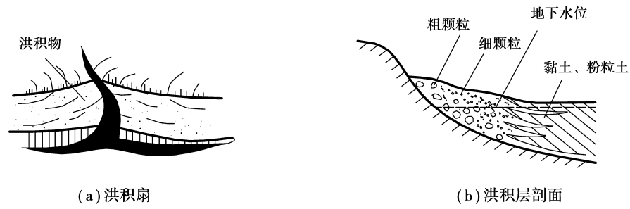
图 1.3 洪积土
