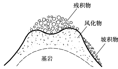
图 1.1 残积土
