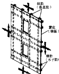
图 1.1.12 应力蒙皮结构局部示意
