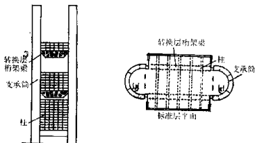
图 1.1.7 华侨银行大楼结构示意图
