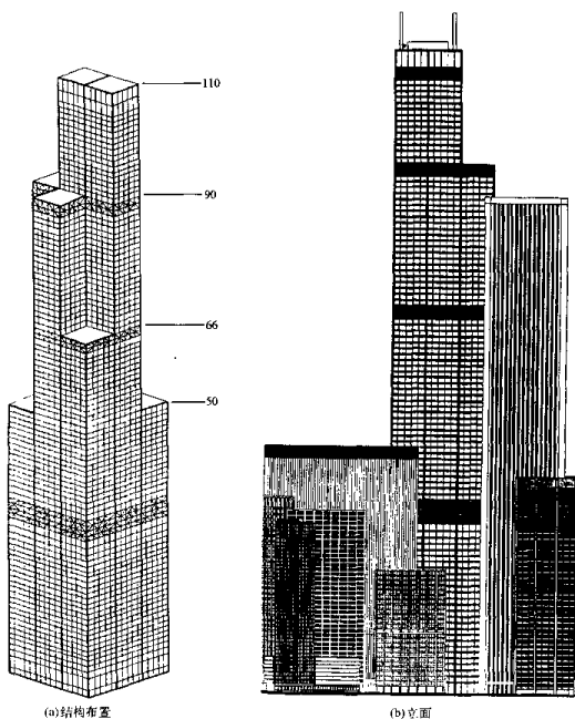
图 1.1.2 西尔斯大厦
