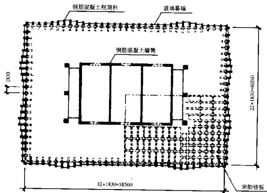
图 1.1.8 贝壳广场大厦平面
