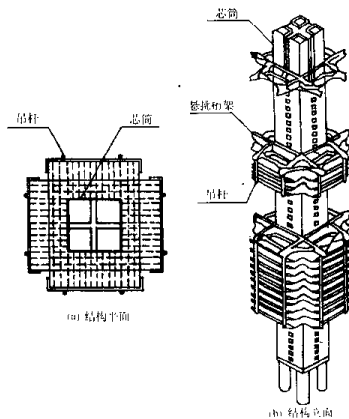
图 1.1.1 标准银行大楼结构示意图
