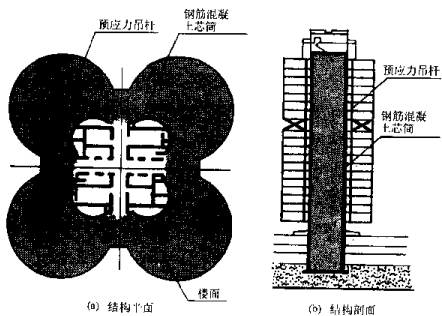
图 1.1.5 桑元里广播中心
