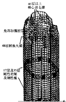
图 1.1.13 One Mellon 银行中心上部楼层骨架(已除去表面蒙皮)
