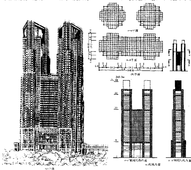
图 1.1.10 东京都府大厦
