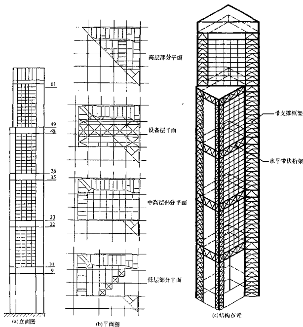
图 1.1.11 新加坡海外联合银行大楼
