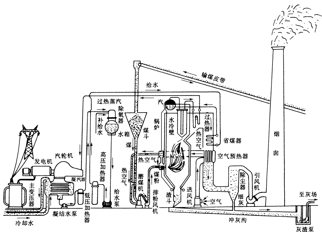
图 0-1 火力发电厂生产过程示意
