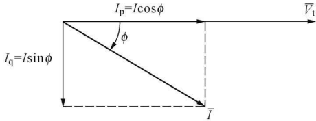
图 1.1 同相和正交的电流分量
