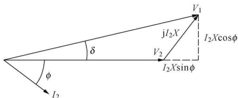
图 1.4 图 1.3 互联的相量图
