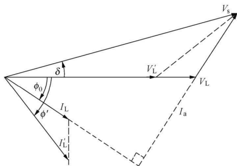
图 1.5 负荷功率因数对负荷端电压的影响
