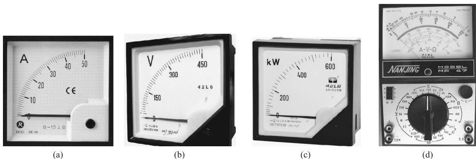
图 1-1 电工仪表的面板示例
