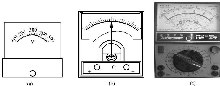
图1-9 指示仪表
