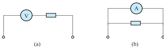
图 1-5 测量线路
