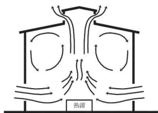
图1-2 热压通风示意
