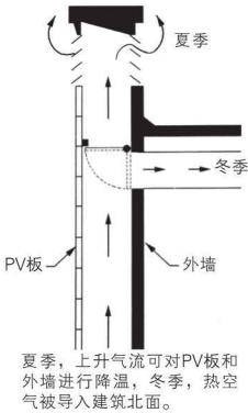
图1-4 透明材料加墙体的双层表皮
