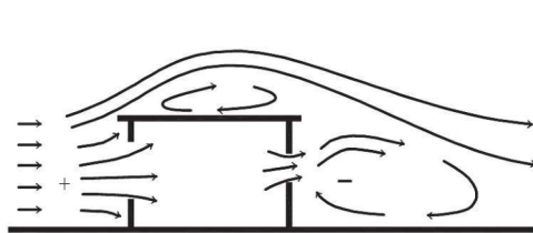
图1-1 风压通风示意
