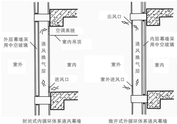
图1-5 呼吸式双层幕墙
