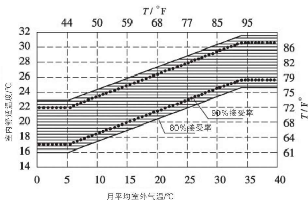
图1-6 自然通风热舒适适应性模型
