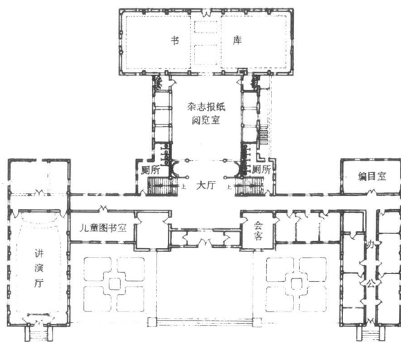
1935年建成的上海市立图书馆立面图与平面图
